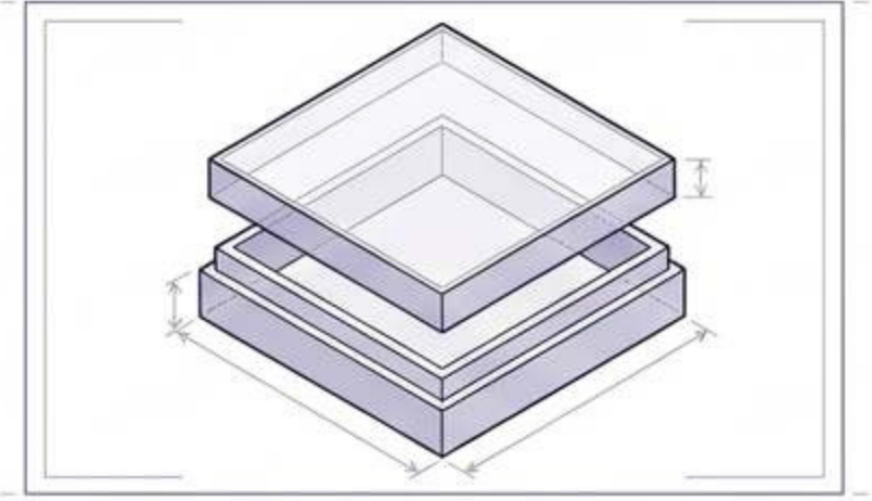
Kapak ve Taban Kutuları (Yalnızca rijit Acrylic için)
