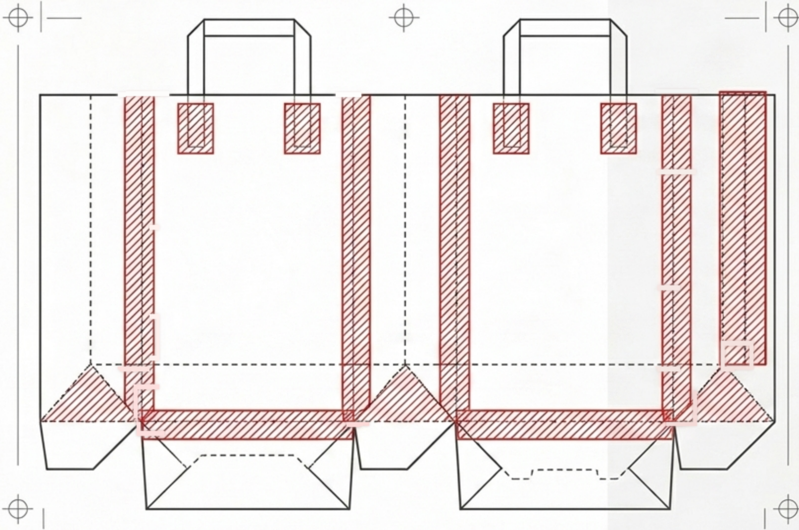
Düzleştirilmiş kalıp çizimi
